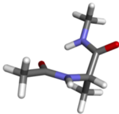
(b) 生成物
